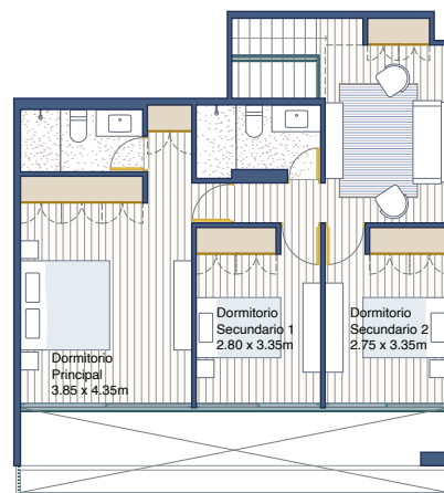
Segunda planta
