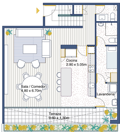
Primera planta
